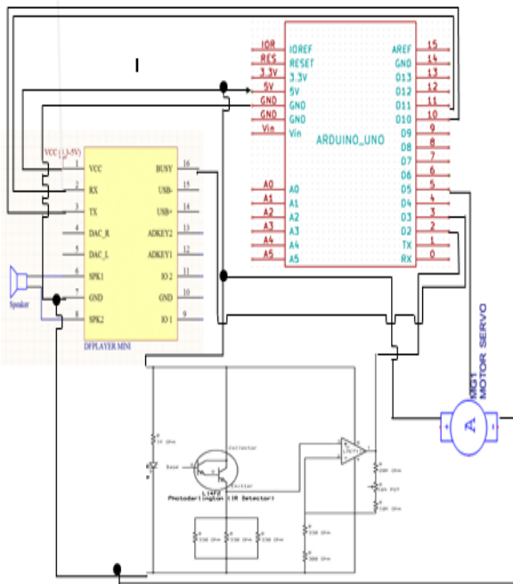
Gambar 6. Rangkaian Keseluruhan Sistem
